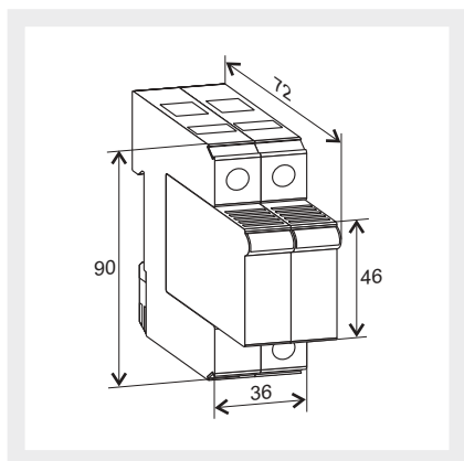
Jednofazowa sieć TT (1+1)
